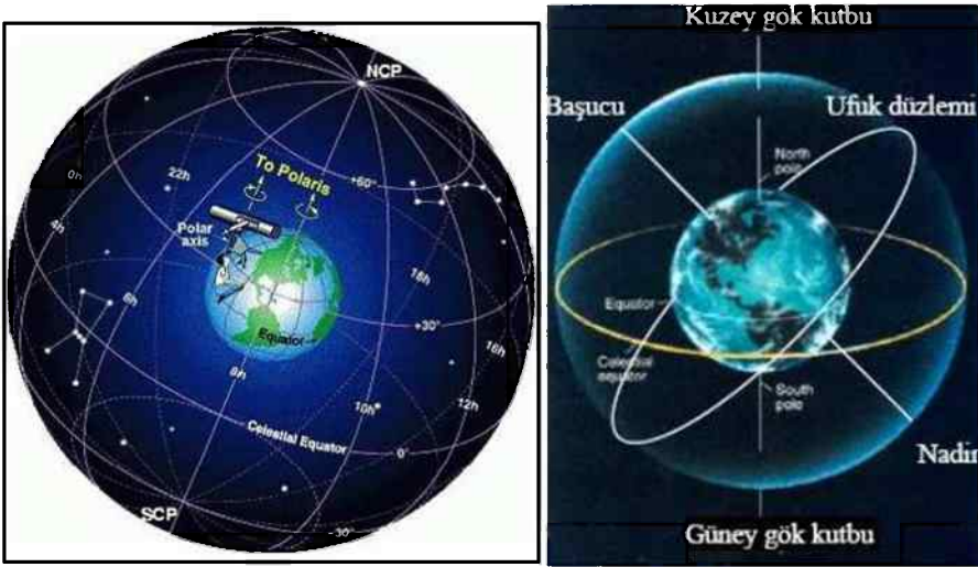
Şekil 1. Gök küresi.
