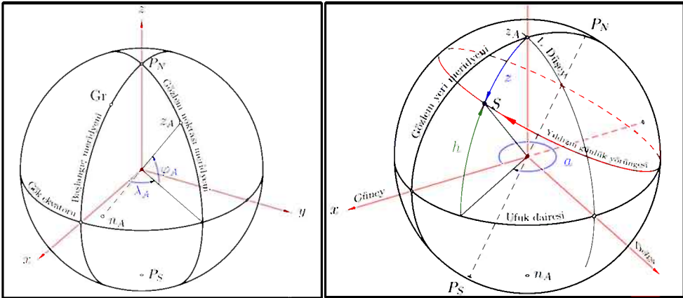
Şekil 2. Enlem ve boylam daireleri.
