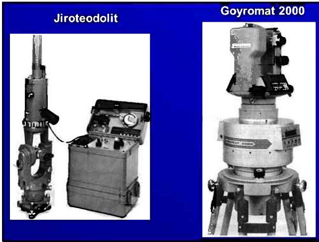
Şekil 14. Jiroskop.
