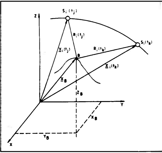
Şekil 5. Uydu jeodezisinde geometrik ilişki (Seeber,1993).
