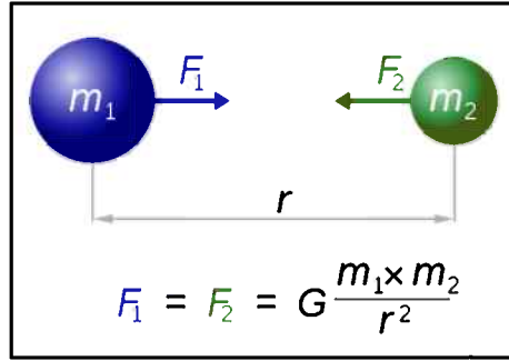
Şekil 1. Evrensel kütle çekimi yasası.
