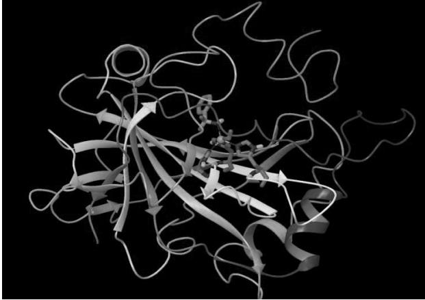
Şekil 2. İnsan karbonik anhidraz II enziminin üç boyutlu (tersiyer) yapısı 33 .
