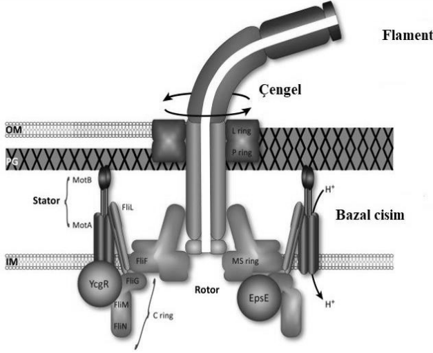
Şekil 1. Bakteri kamçısının genel yapısı 65 .
