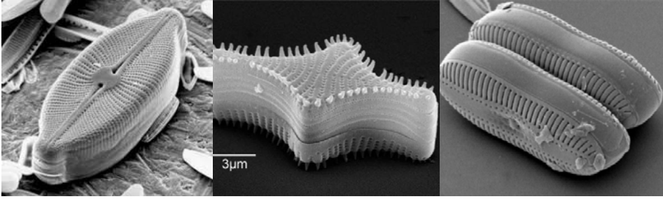
Şekil 4. Pennat Diyatomeler
