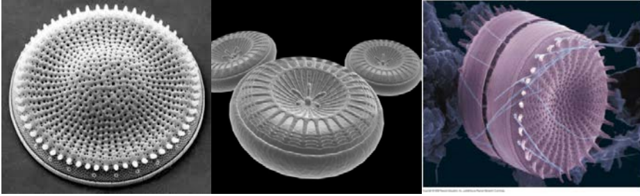
Şekil 3. Sentrik diyatomeler
