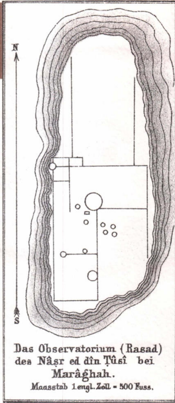
Houtum-Schindler'e göre Merāġa Rasathanesi'nin yatay izdüşümü (1270 civarı).
