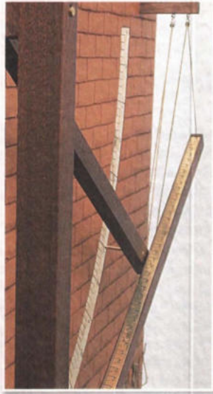
Modelimiz: Ahşap, astarlanmış; mermer kaide. Kadran pirinçten, asitle derecelendirilmiş; yarıçap: 40 cm. Cetveller tik ağacından iki direk arasında dikey olarak hareket edebilir. Yükseklik 64 cm. Kiriş cetveli üzerinde metrik ölçek bulunmaktadır. (Envanter No: A 4.26)
