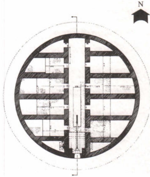
Merkezi kulenin sekstantla birlikte yatay izdüşümü.
