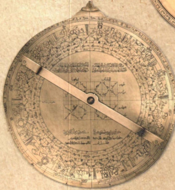
1. ve 2. Resim Modelimiz: Piring, hâkkedilmiş; Ø = 560 mm. (Envanter No: A 2.24)
