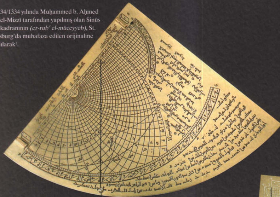
Pirinç, hâkkedilmiş. Yarıçap 150 mm. Ön yüz nişangâhlı. (Envanter No: A 3.03)
