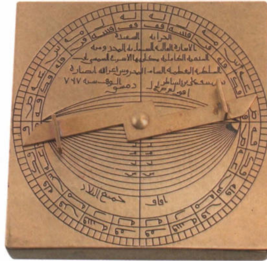
Modelimizin dış görünüşü (usturlap).
