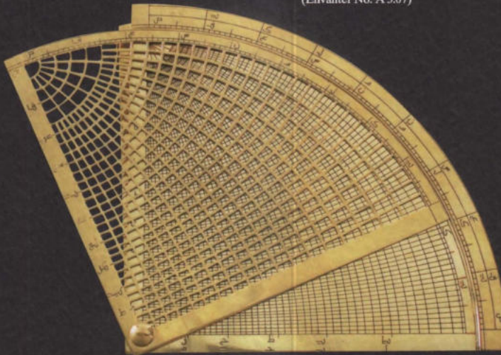
Pirinç, hâkkedilmiş. Yarıçap 167 mm. (Envanter No: A.3.07)
