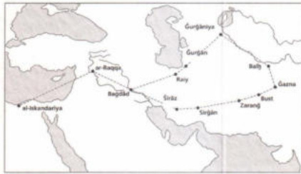
4. Resim: el-Birûnî tarafından 11. yüzyılın ilk çeyreğinde arşınlanan mesafeler ve astronomik olarak ölçülen enlemler vasıtasıyla Bağdat ile Gazne arasındaki yaklaşık 60 yerin boylam derecelerini hesaplamaya yönelik yapılan çalışmanın şematik sunumu.
