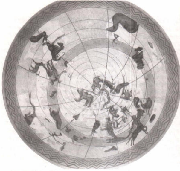
Kūshayr 'Amra Roma Hamamı (Caldarium)'nın kubbesindeki gök haritasının rekonstrüksiyonu (M. Stein).
