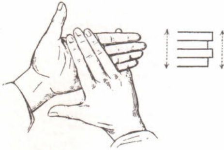
Bir zübân'ın =4 işba' el parmaklarıyla belirlenmesi (Léopold de Saussure'e göre)
