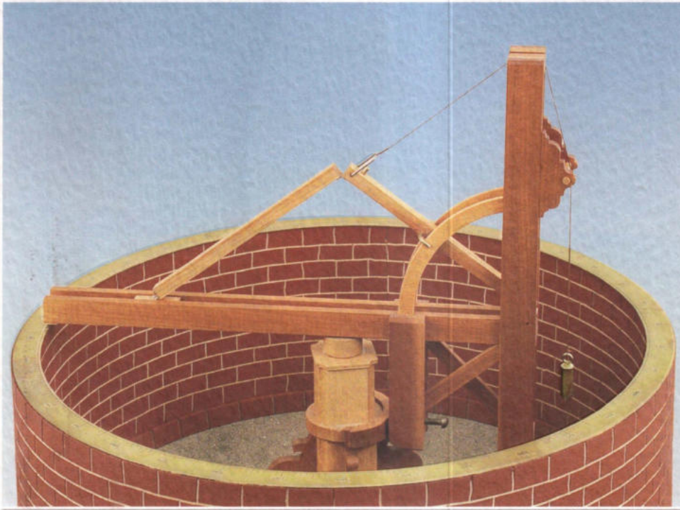
Ölçek 1:10. Çap 50 cm. Başlık ahşap, eksensel döndürülebilir. Bacak bir karşı ağırlıkla kolayca döndürülmekte. Derece taksimatlı pirinç skala. (Envanter No: A 4.08)
