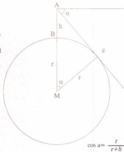
Dünya yarıçapının Sind b. 'Alî tarafından hesaplanma yöntemi.
