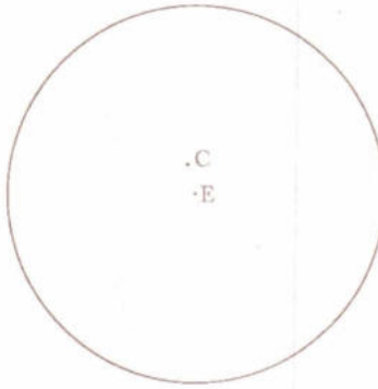
E = Dünya'nın merkezi C = Eksantrik dairenin veya deferentin merkezi
