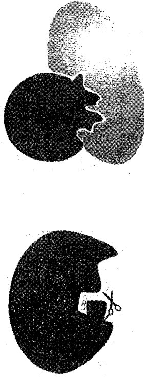
Şekil 3-1: (Üstte) İki protein bağlandığı zaman şekilleri birbirine oldukça uyumludur. (Alta) Kimyasal bir tepkimeyi katalizlemek için bir enzim bağlayacağı gruplara yaklaşır. Makas, bir molekülü kimyasal olarak kesen bir proteini temsil eder ve şekilde açık renkle gösterilmiştir.
