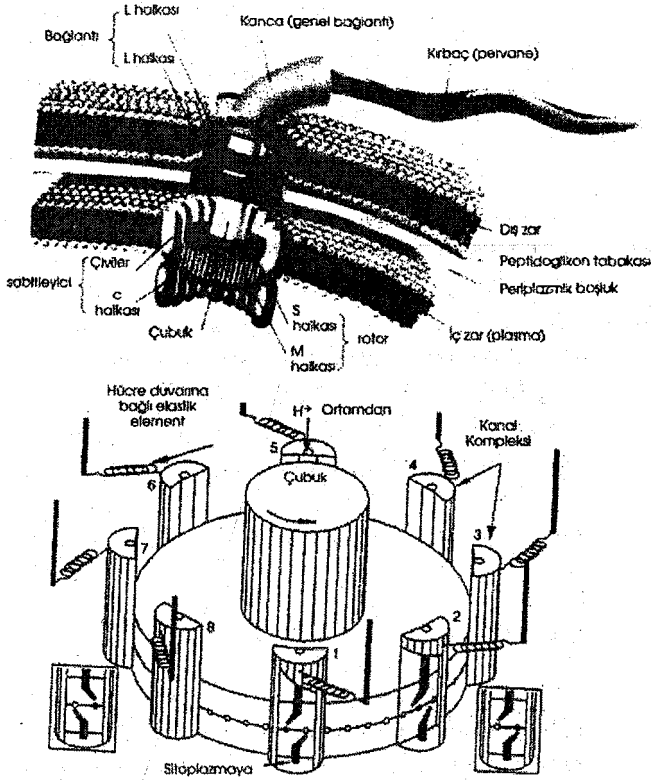
Şekil 3-3: (Üstte) İç ve dış hücre zarı ile hücre duvarına gömülü iplik, askı ve motoru gösteren bir bakteri kamçı şekli. (Alta) Asit güdümlü dönme motoru için önerilen bir model. Şekil, motorun kitapta ele alınmayan iç karmaşıklığını göstermektedir.
